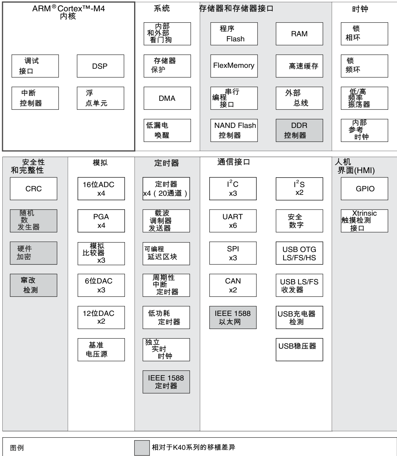
图 2. K60 框图
