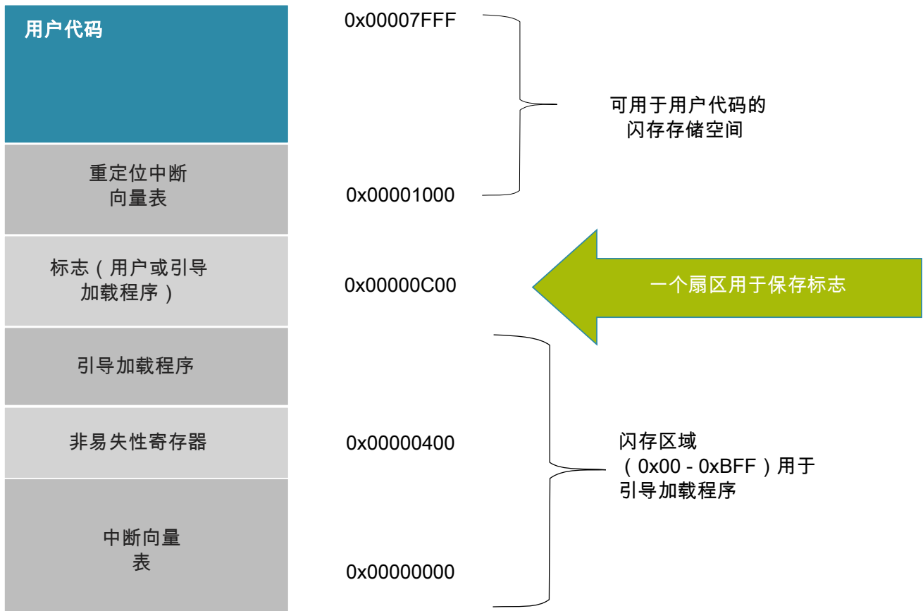
图 5. 存储器分配
